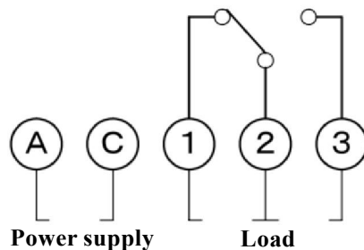
▲ Nối dây
